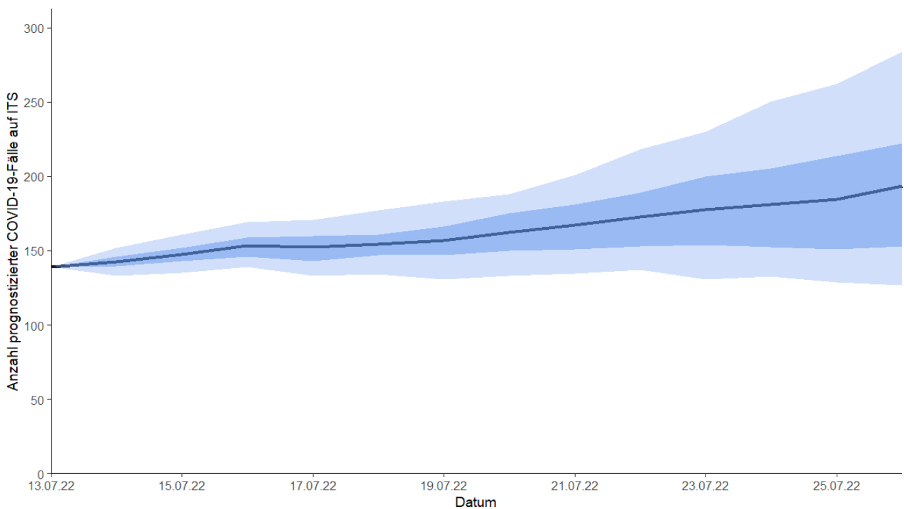
Abbildung 12: Anzahl prognostizierter COVID-19 Fälle auf ITS nach Datum ab dem 13.07.2022 für 14 Tage mit Interquartilsabstand (dunkel) und 95%-Vorhersageintervall (hell), Baden-Württemberg, Stand RKI und DIVI-Intensivregister ( www.intensivregister.de ): 14.07.2022, 15:30 Uhr. (Quelle: Berechnungen auf der Basis des Modells des Instituts für Infektionsprävention und Krankenhaushygiene, Universitätsklinikum Freiburg)
